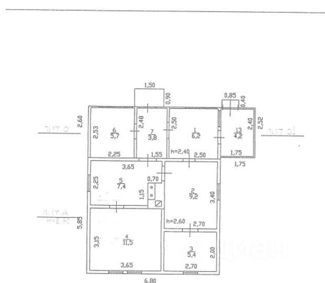
6. Поэтажный план
