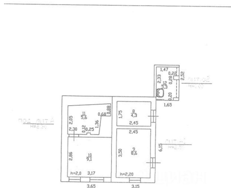
6. Поэтажный план
