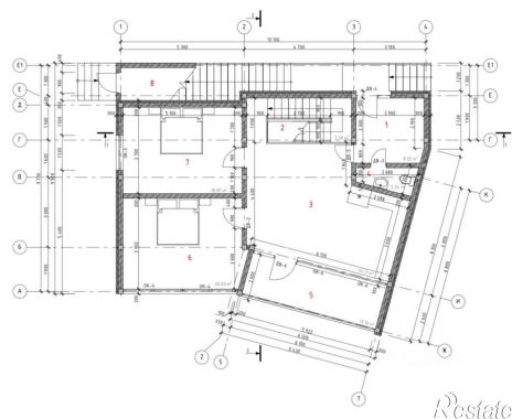
План 2 этажа
