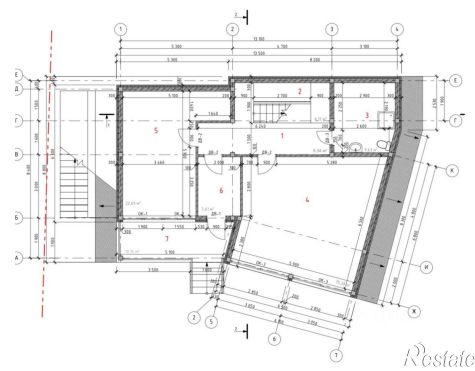
План 1 этажа
